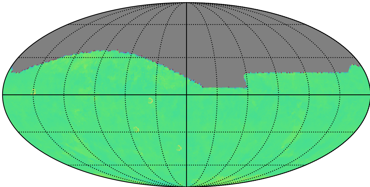
noroll_mjdp120_v3.4_10yrs r: Kuiper rotTelPos
