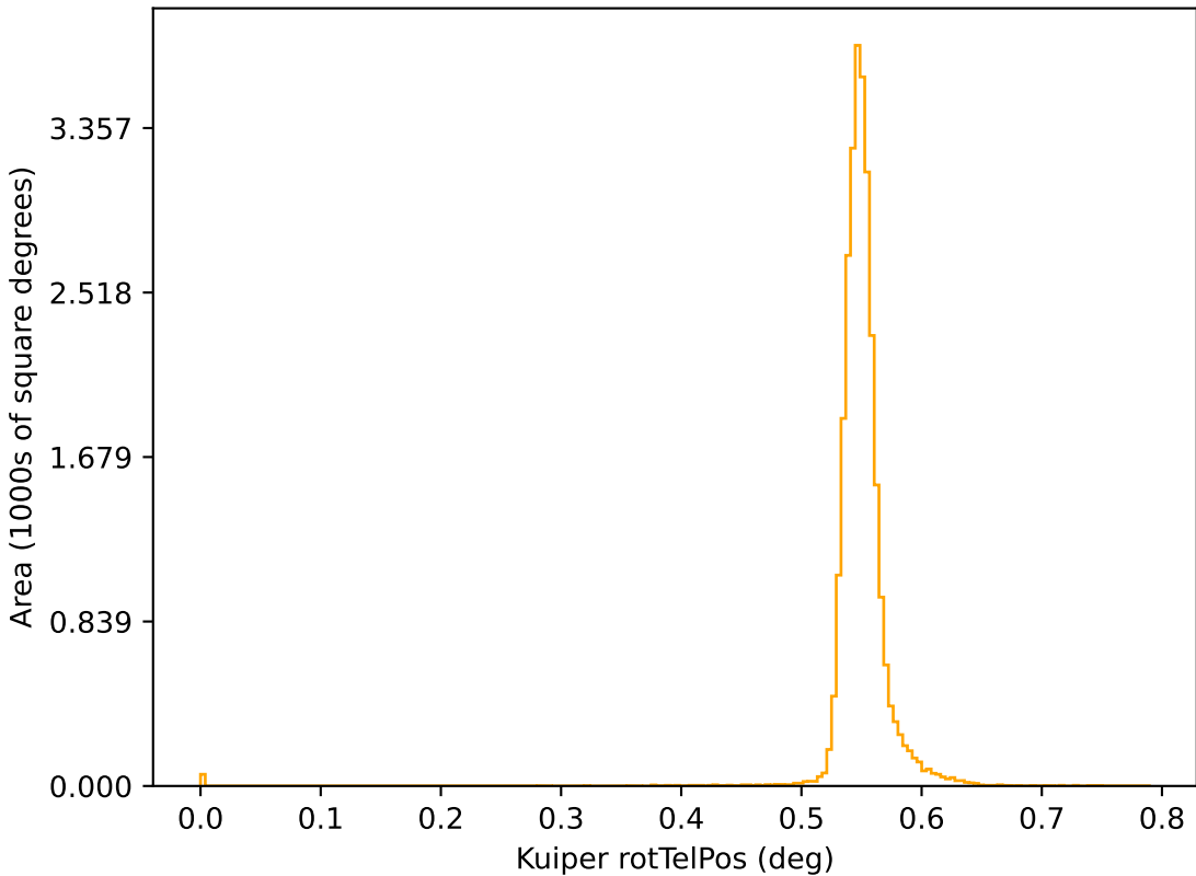
noroll_mjdp120_v3.4_10yrs r: Kuiper rotTelPos
