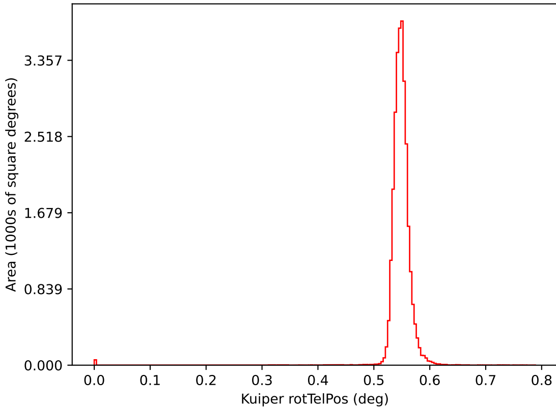
noroll_mjdp120_v3.4_10yrs i: Kuiper rotTelPos
