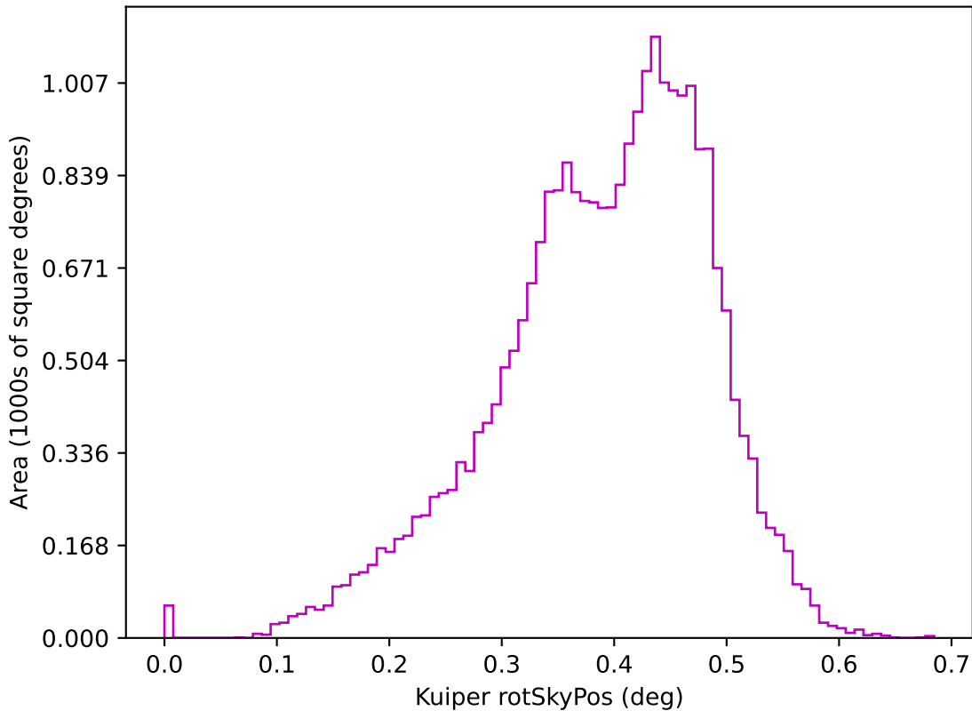
noroll_mjdp120_v3.4_10yrs z: Kuiper rotSkyPos
