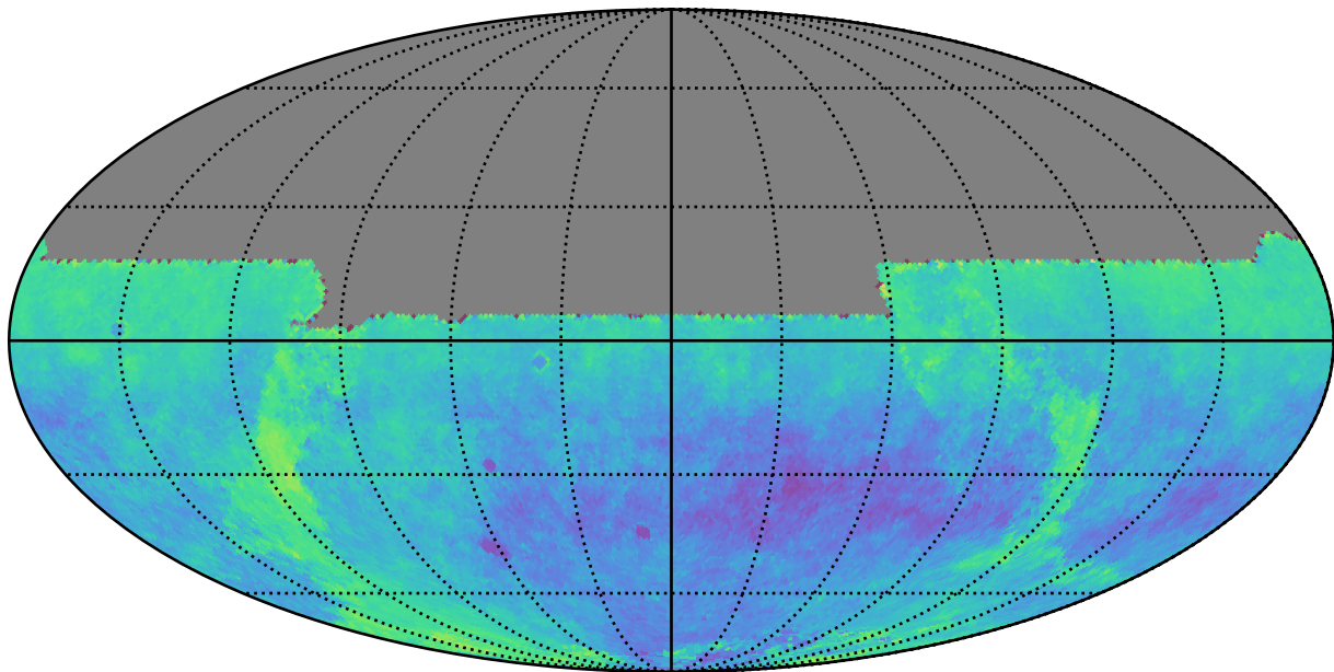
noroll_mjdp120_v3.4_10yrs y: Kuiper rotSkyPos
