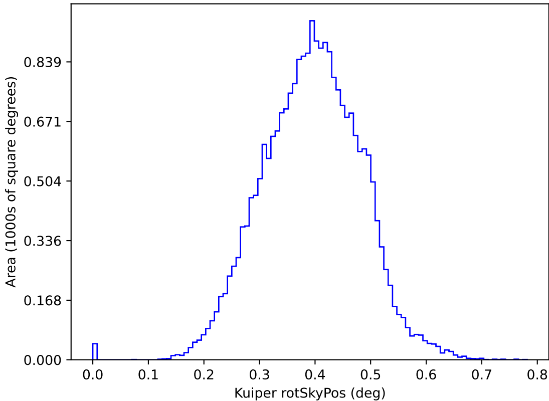
noroll_mjdp120_v3.4_10yrs y: Kuiper rotSkyPos
