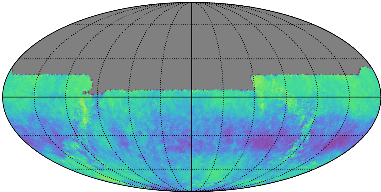
noroll_mjdp120_v3.4_10yrs u: Kuiper rotSkyPos
