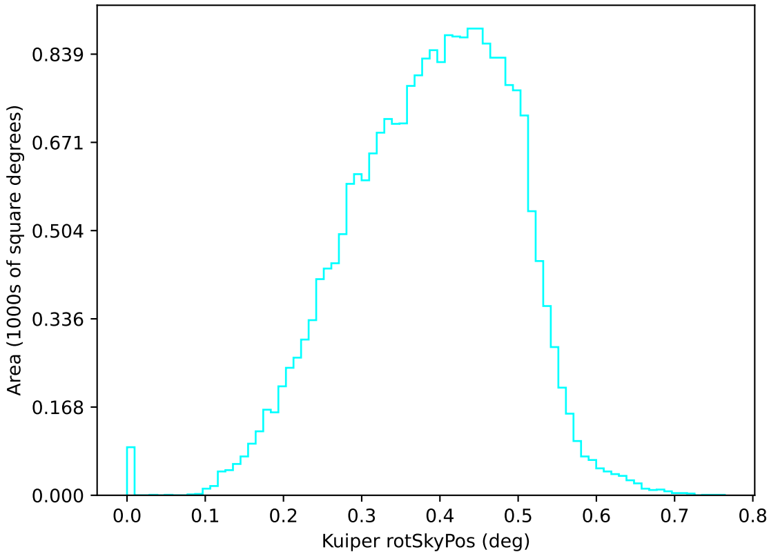
noroll_mjdp120_v3.4_10yrs u: Kuiper rotSkyPos
