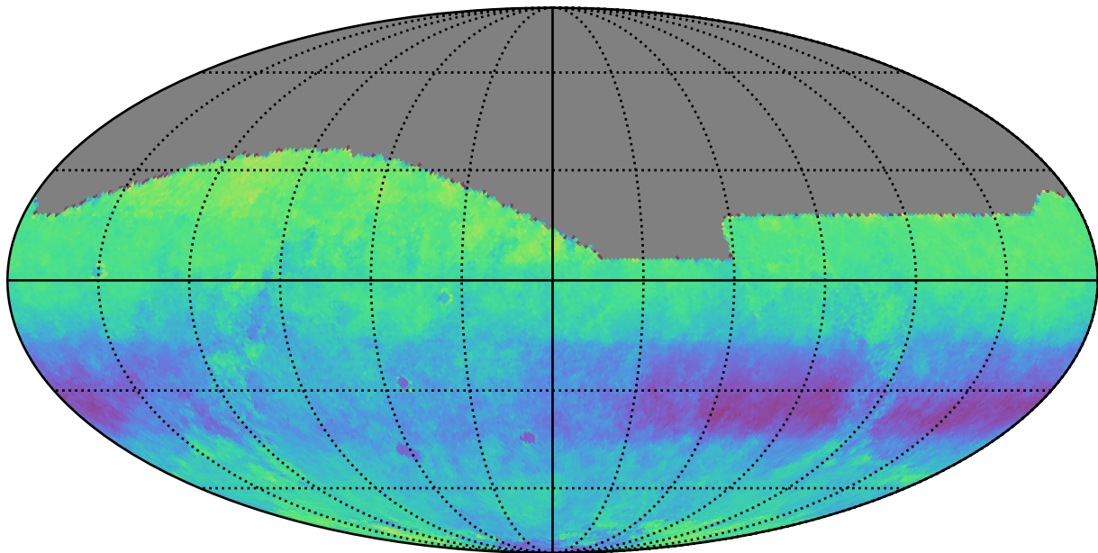
noroll_mjdp120_v3.4_10yrs r: Kuiper rotSkyPos
