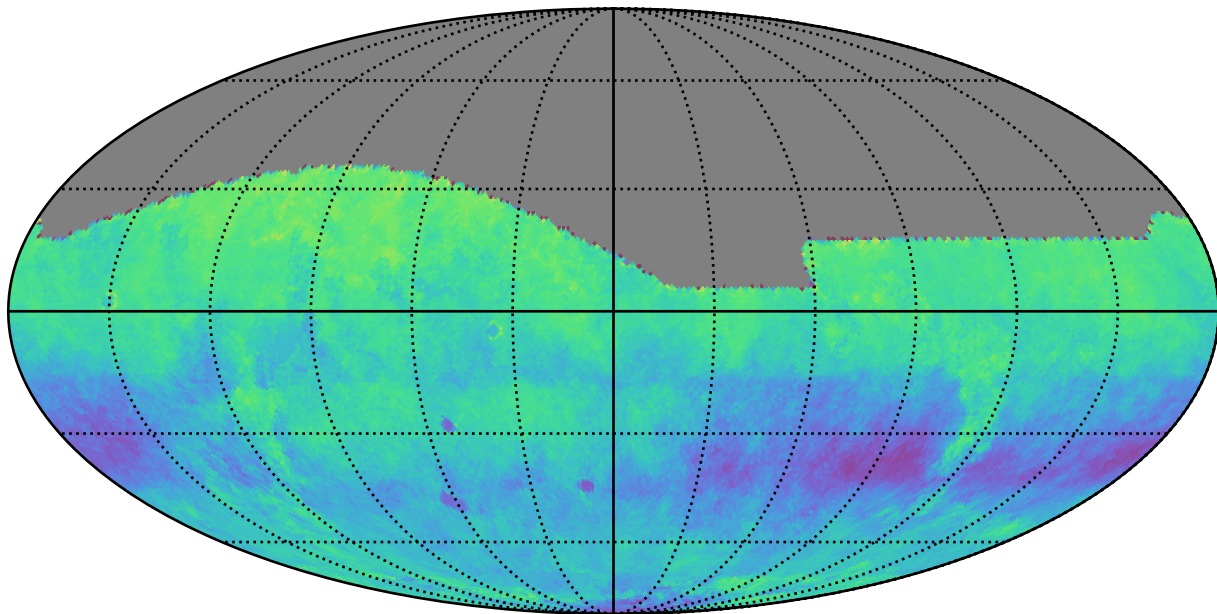
noroll_mjdp120_v3.4_10yrs i: Kuiper rotSkyPos
