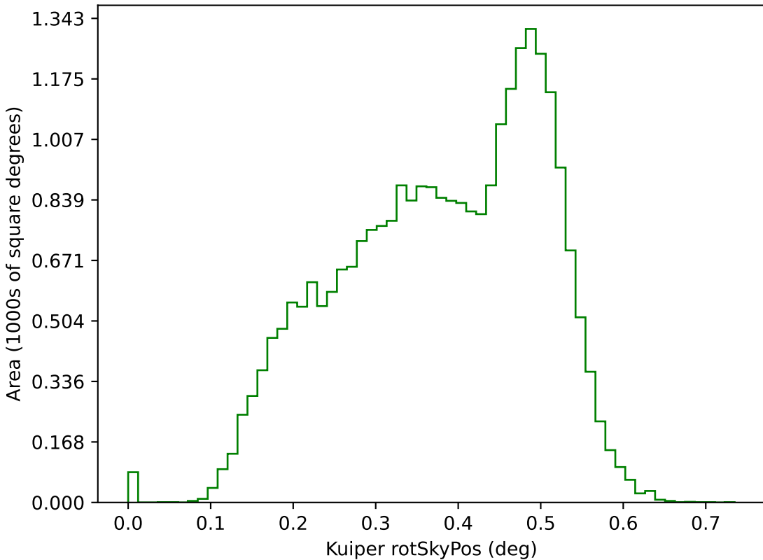
noroll_mjdp120_v3.4_10yrs g: Kuiper rotSkyPos
