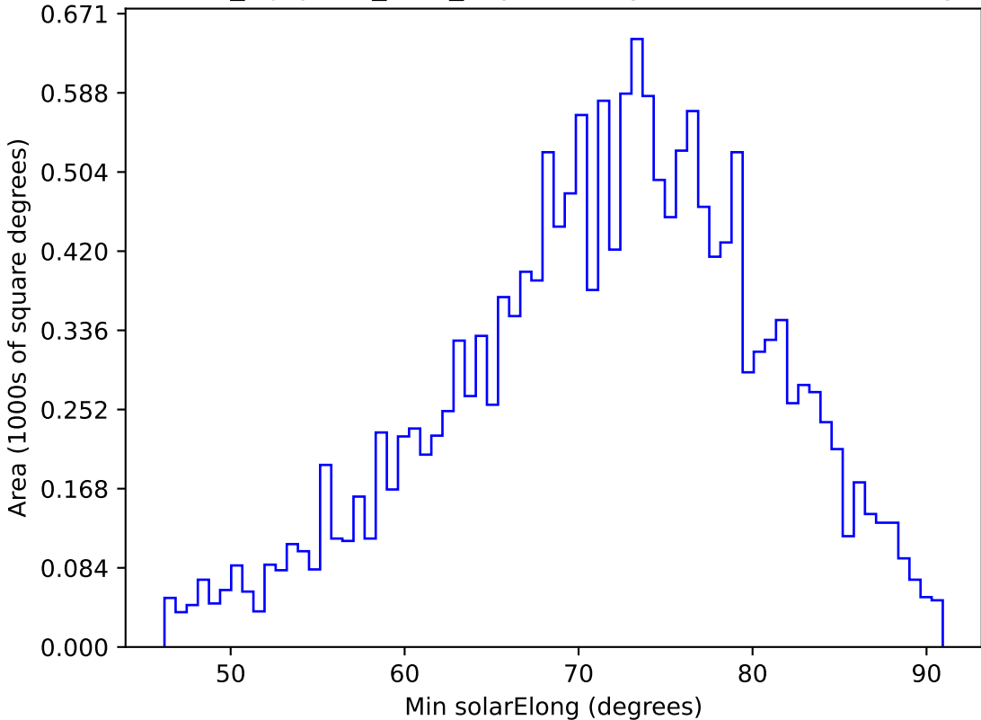
noroll_mjdp120_v3.4_10yrs WFD y band: Min solarElong
