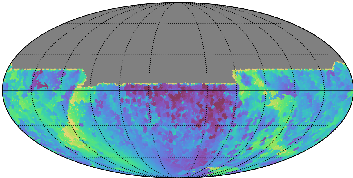
noroll_mjdp120_v3.4_10yrs All sky y band: Min solarElong
