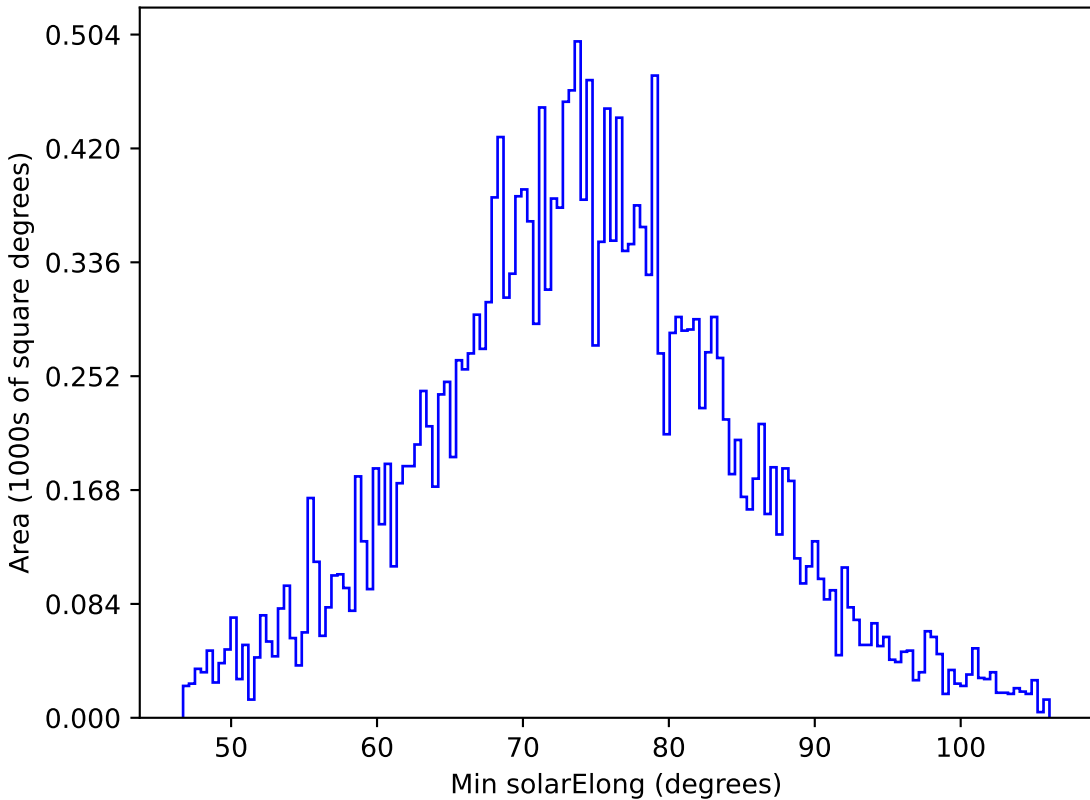
noroll_mjdp120_v3.4_10yrs All sky y band: Min solarElong
