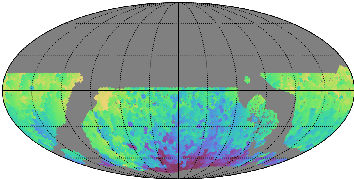
noroll_mjdp120_v3.4_10yrs WFD y band: Min HA
