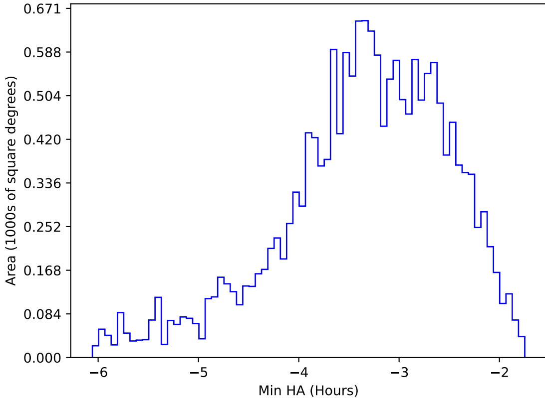
noroll_mjdp120_v3.4_10yrs WFD y band: Min HA
