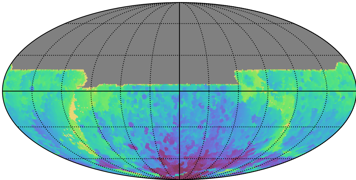
noroll_mjdp120_v3.4_10yrs All sky y band: Min HA
