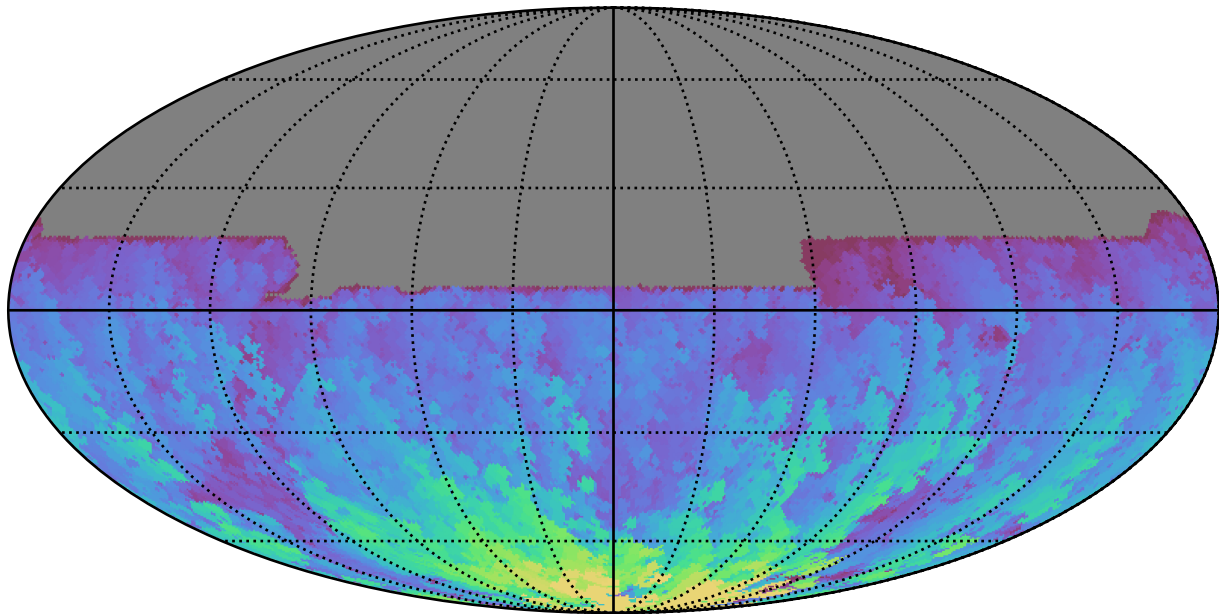
noroll_mjdp120_v3.4_10yrs All sky y band: Max HA
