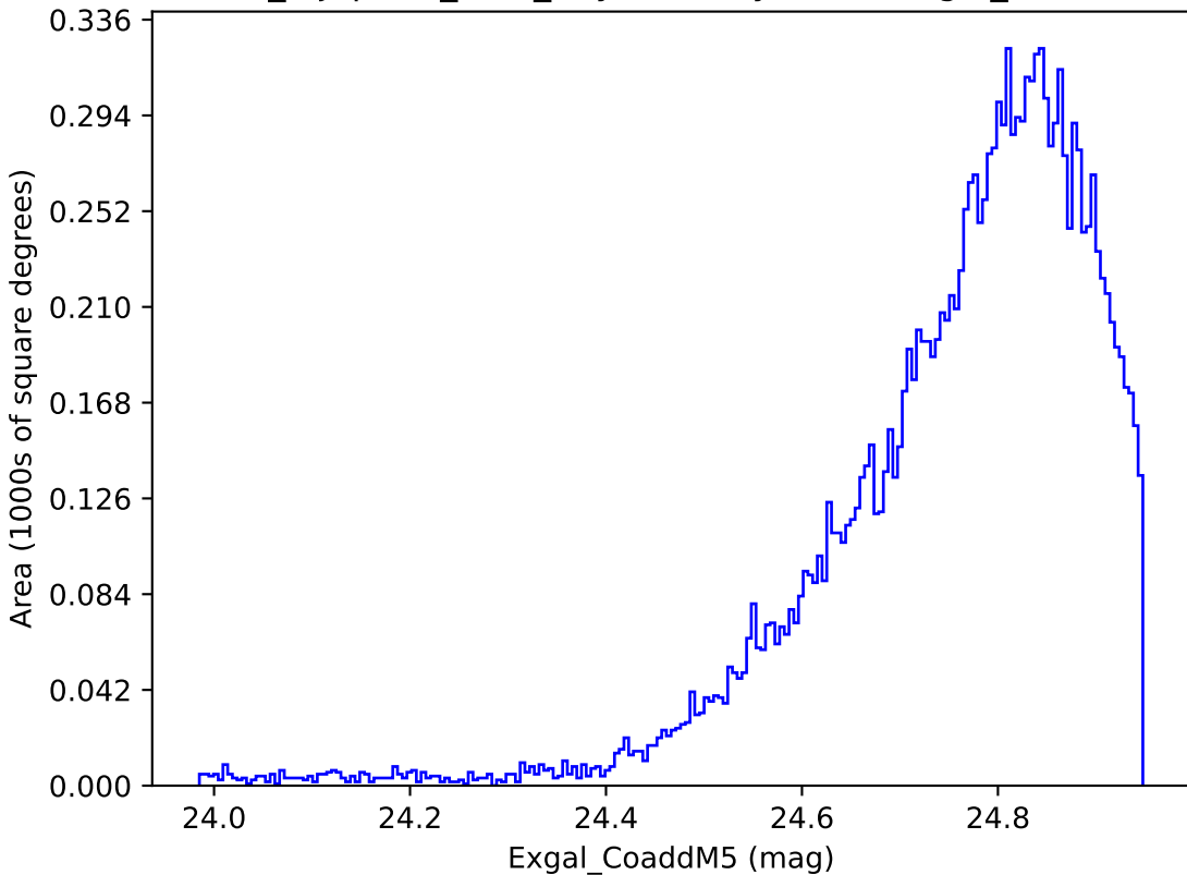
noroll_mjdp120_v3.4_10yrs WFD y band: Exgal_CoaddM5
