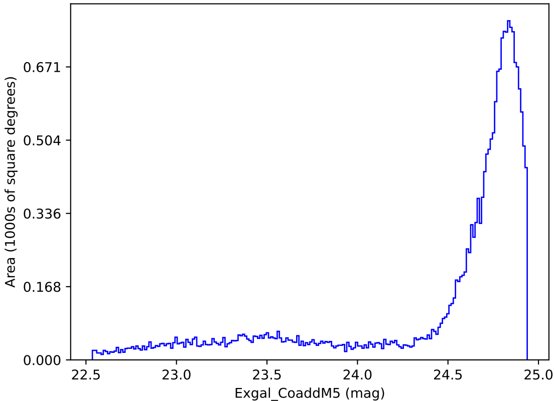
noroll_mjdp120_v3.4_10yrs All sky y band: Exgal_CoaddM5
