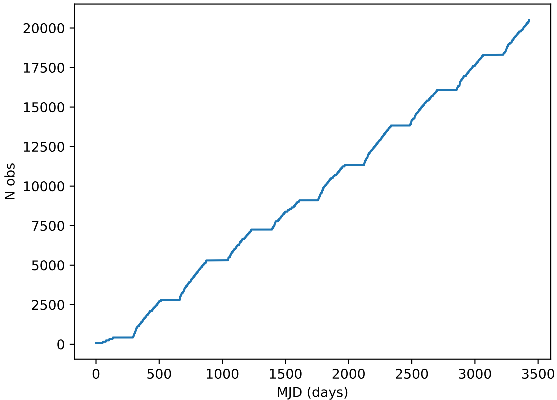
noroll_mjdp120_v3.4_10yrs note like DD:ELAISS1%: Cumulative
