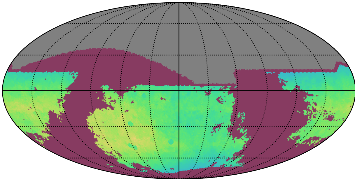
noroll_mjdp0_v3.4_10yrs i: NgalScale
