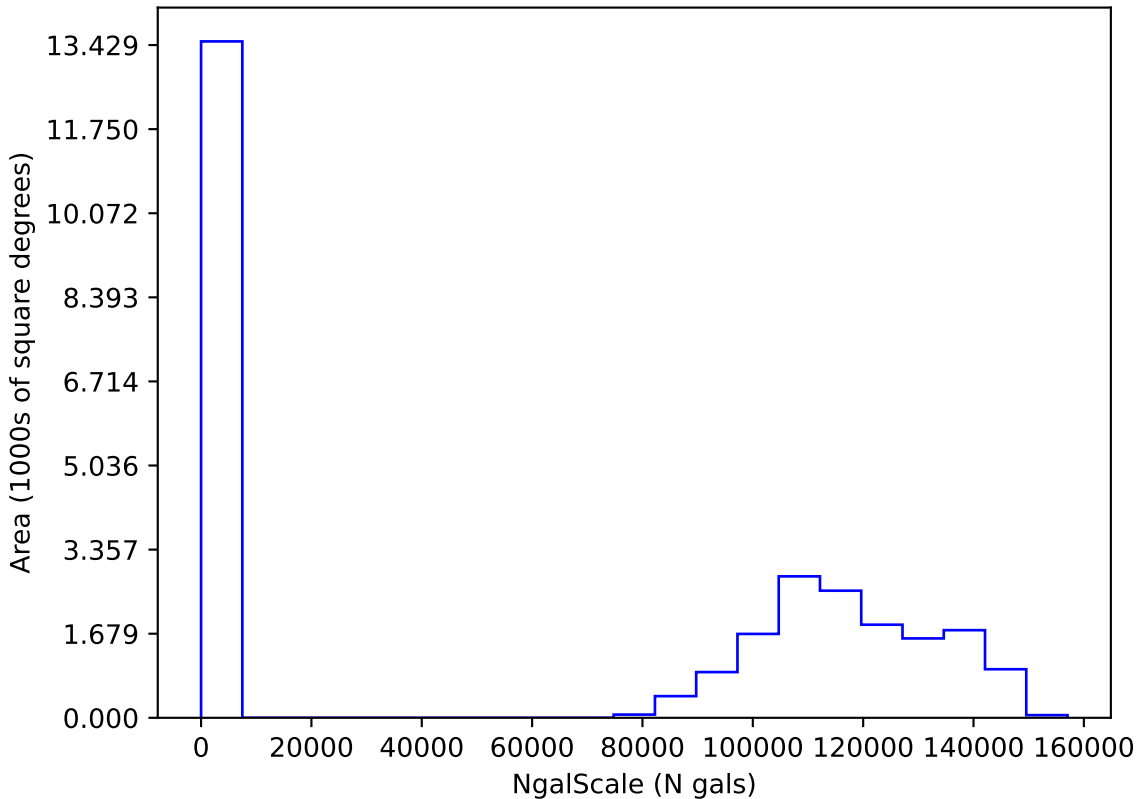
noroll_mjdp0_v3.4_10yrs i: NgalScale
