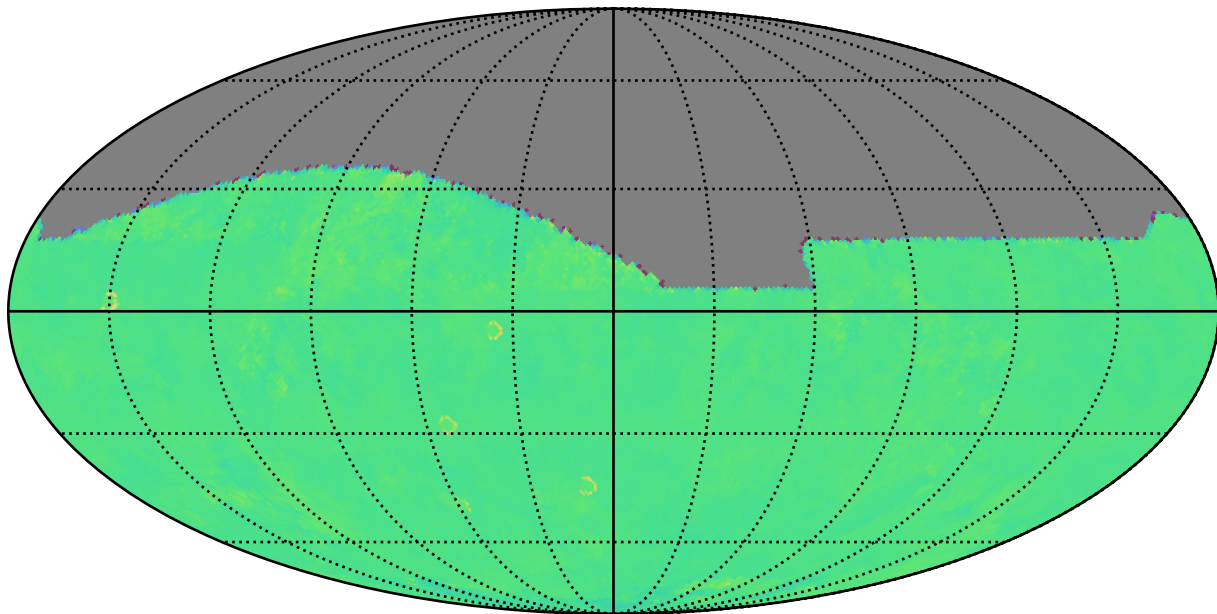
noroll_mjdp0_v3.4_10yrs z: Kuiper rotTelPos
