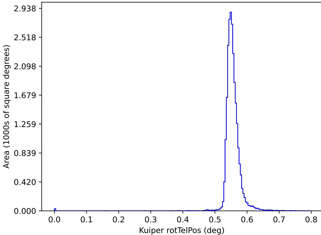
noroll_mjdp0_v3.4_10yrs y: Kuiper rotTelPos
