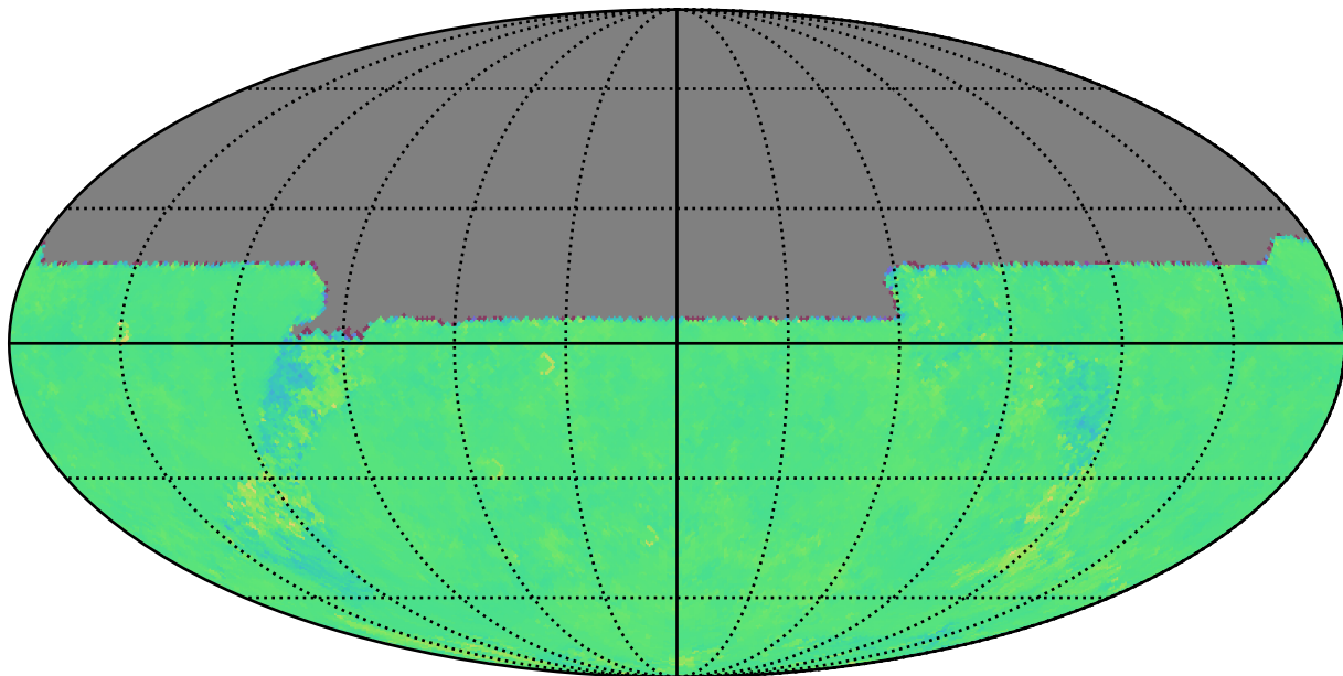
noroll_mjdp0_v3.4_10yrs u: Kuiper rotTelPos
