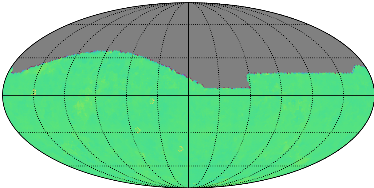
noroll_mjdp0_v3.4_10yrs i: Kuiper rotTelPos
