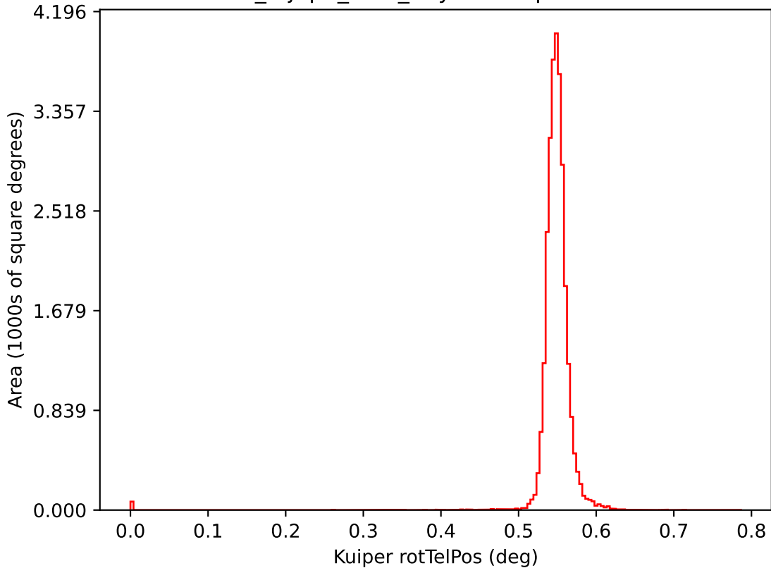
noroll_mjdp0_v3.4_10yrs i: Kuiper rotTelPos
