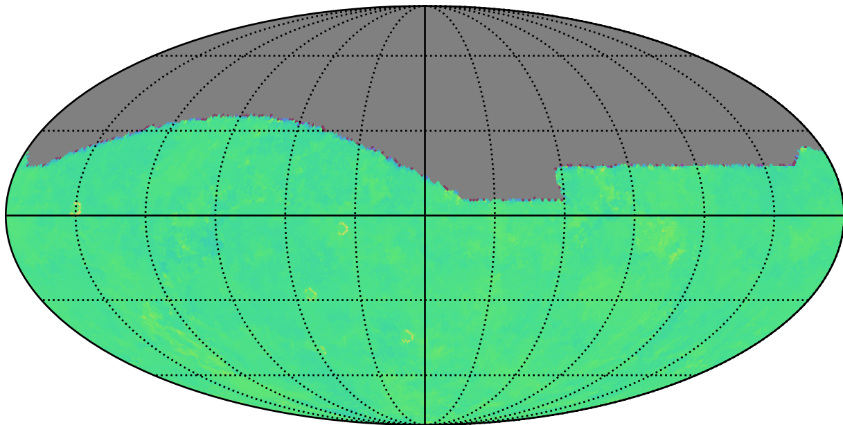
noroll_mjdp0_v3.4_10yrs g: Kuiper rotTelPos
