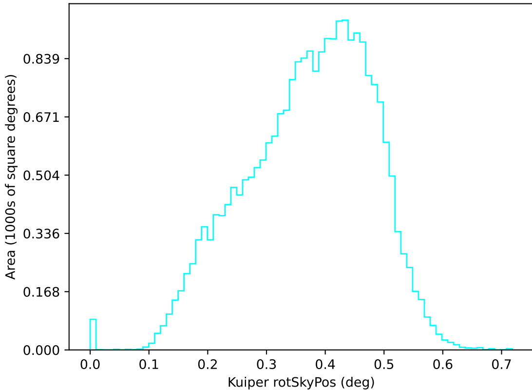
noroll_mjdp0_v3.4_10yrs u: Kuiper rotSkyPos
