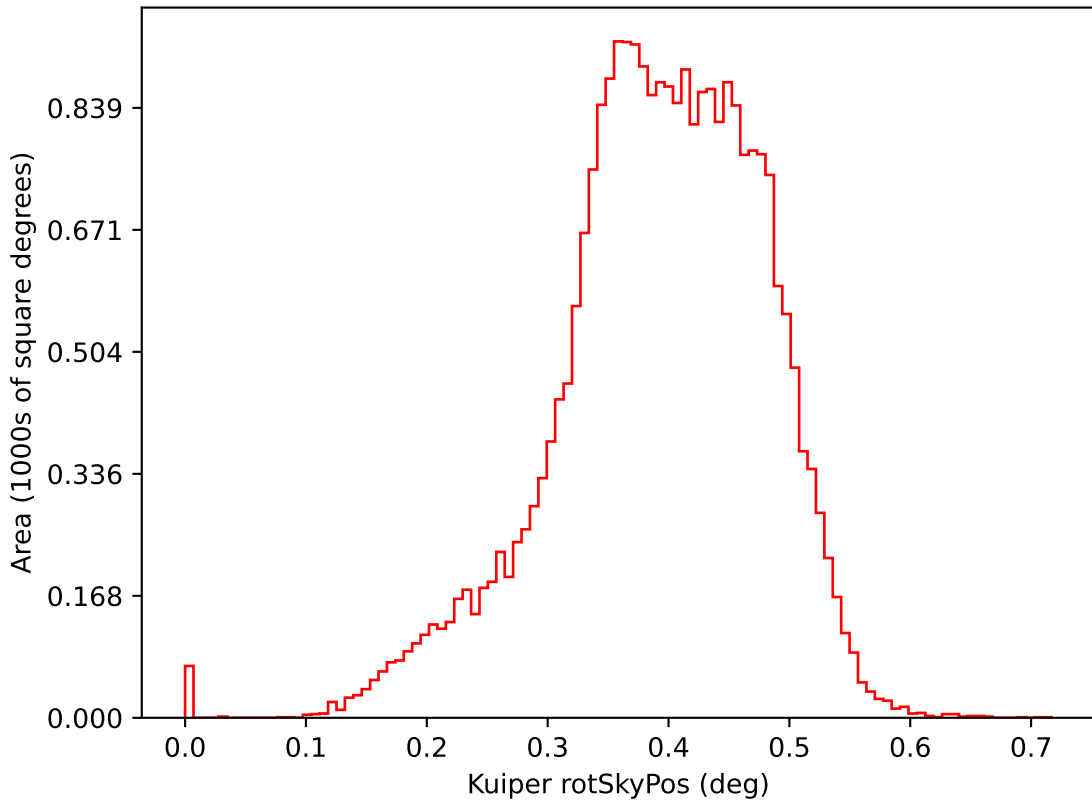
noroll_mjdp0_v3.4_10yrs i: Kuiper rotSkyPos
