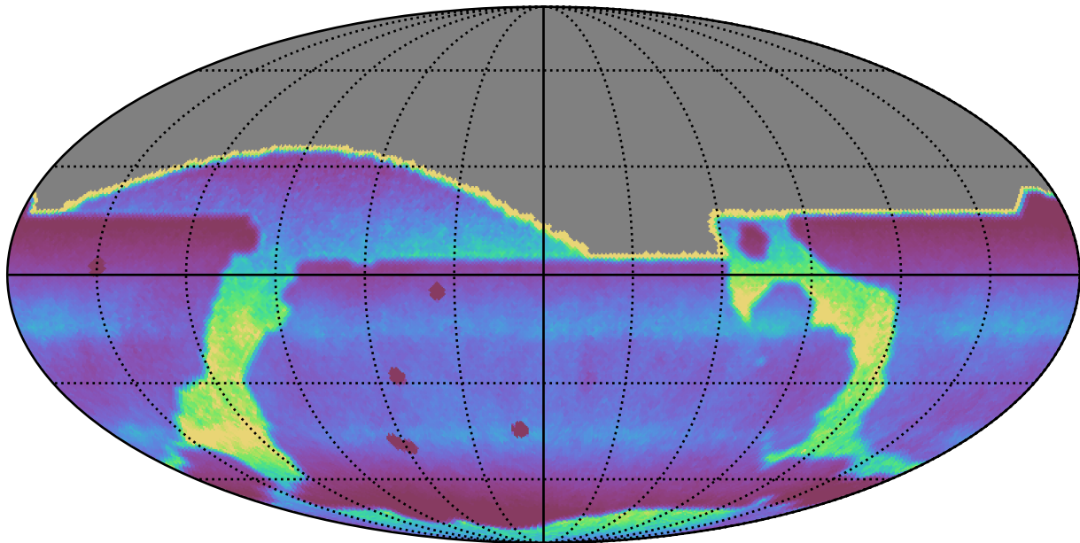
noroll_mjdp0_v3.4_10yrs : DCRprecision
