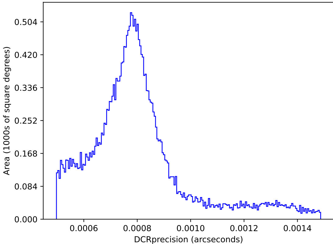
noroll_mjdp0_v3.4_10yrs : DCRprecision
