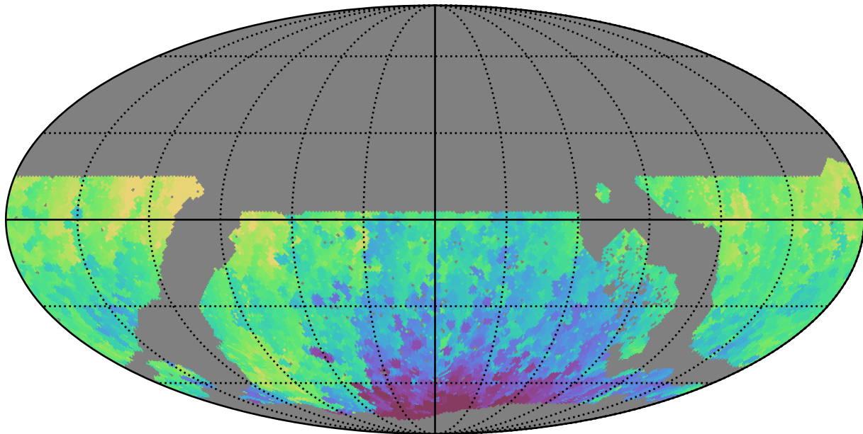
noroll_mjdp0_v3.4_10yrs WFD y band: Min HA
