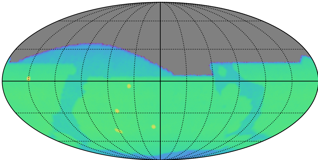
noroll_mjdp0_v3.4_10yrs i: CoaddM5
