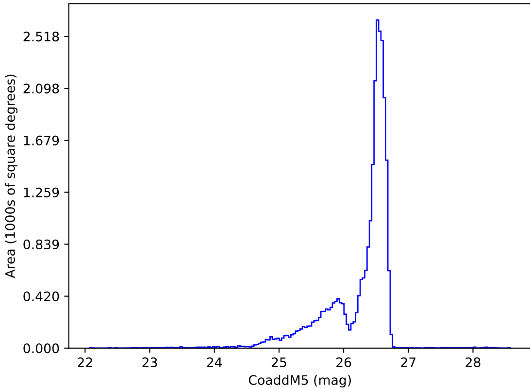
noroll_mjdp0_v3.4_10yrs i: CoaddM5
