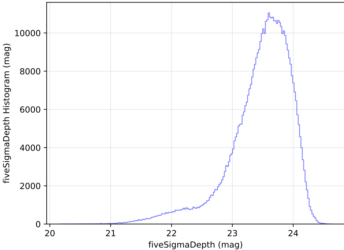
no_magell_roll_v3.4_10yrs i: fiveSigmaDepth Histogram
