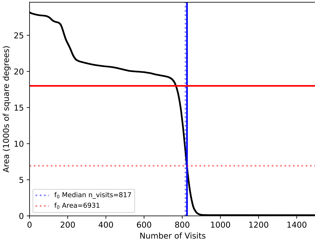
no_magell_roll_v3.4_10yrs : f0
