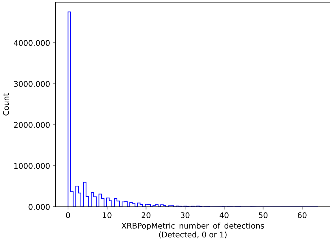
no_magell_roll_v3.4_10yrs : XRBPopMetric_number_of_detections
