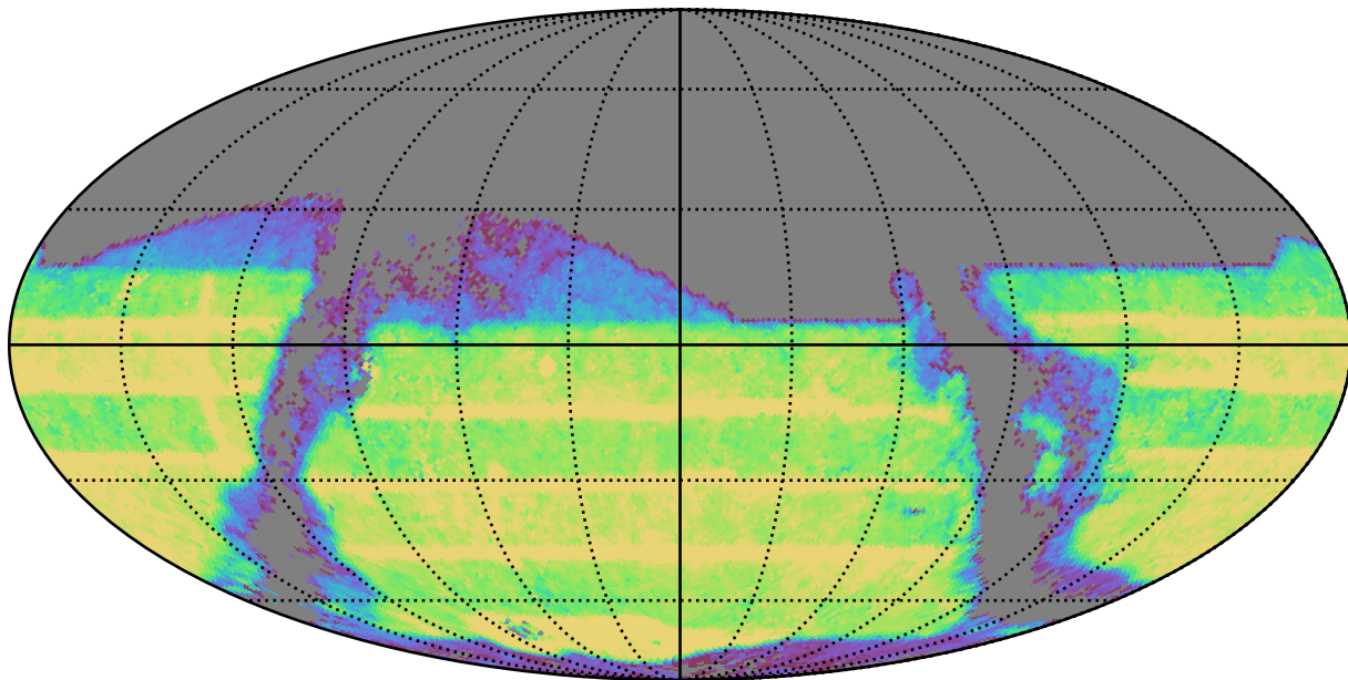
no_magell_roll_v3.4_10yrs : TDC_rate
