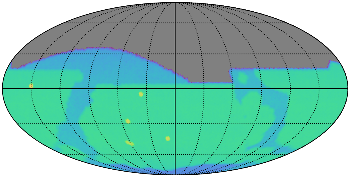
no_magell_roll_v3.4_10yrs i: SurfaceBrightLimit
