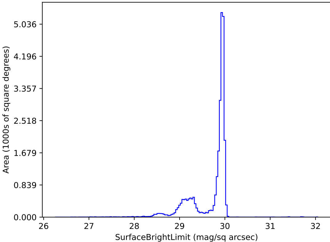
no_magell_roll_v3.4_10yrs i: SurfaceBrightLimit
