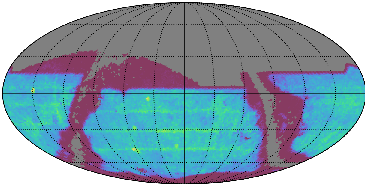
no_magell_roll_v3.4_10yrs : SNSLMetric
