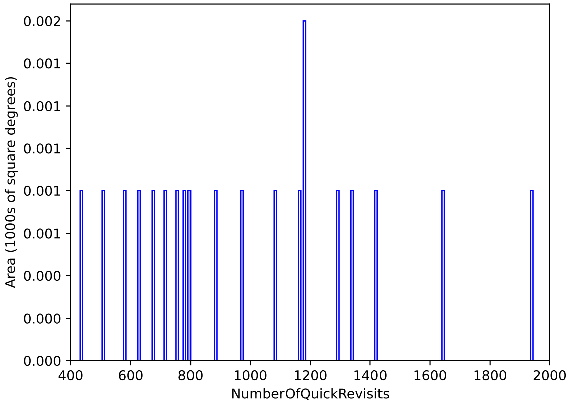
no_magell_roll_v3.4_10yrs : NumberOfQuickRevisits
