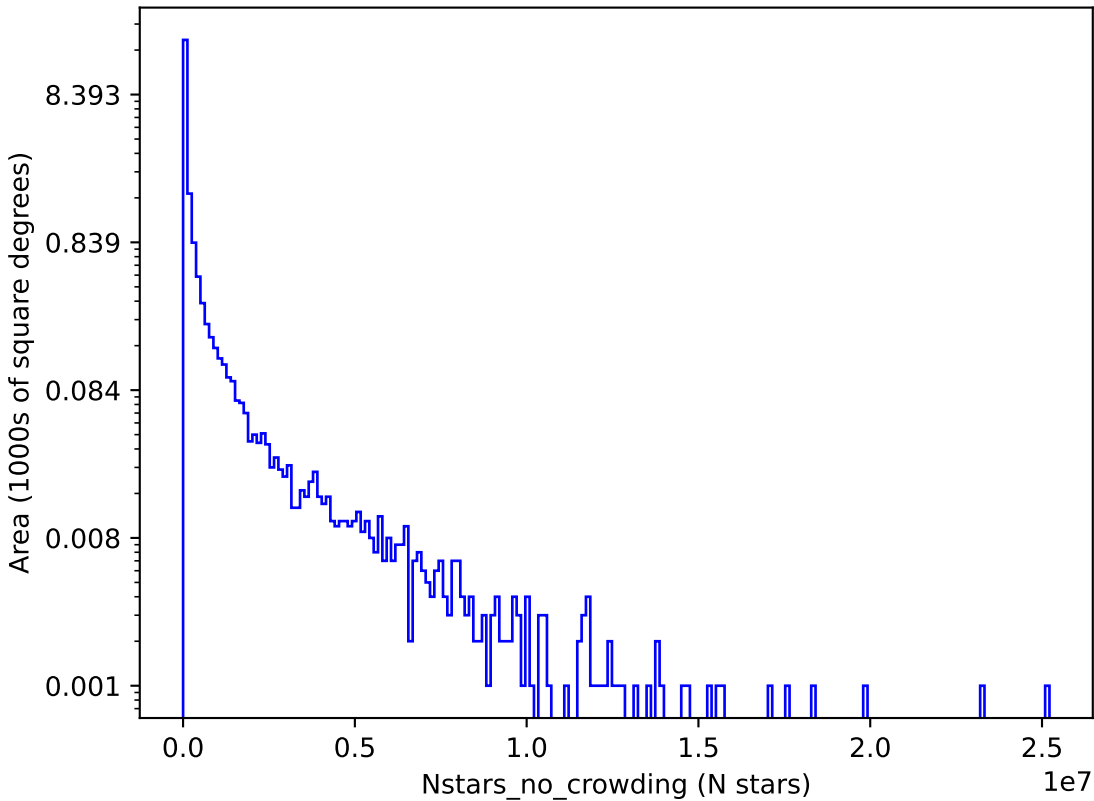
no_magell_roll_v3.4_10yrs y: Nstars_no_crowding
