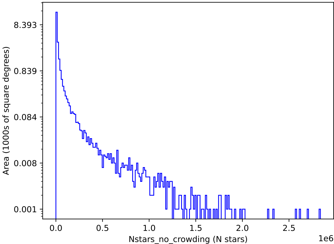
no_magell_roll_v3.4_10yrs u: Nstars_no_crowding
