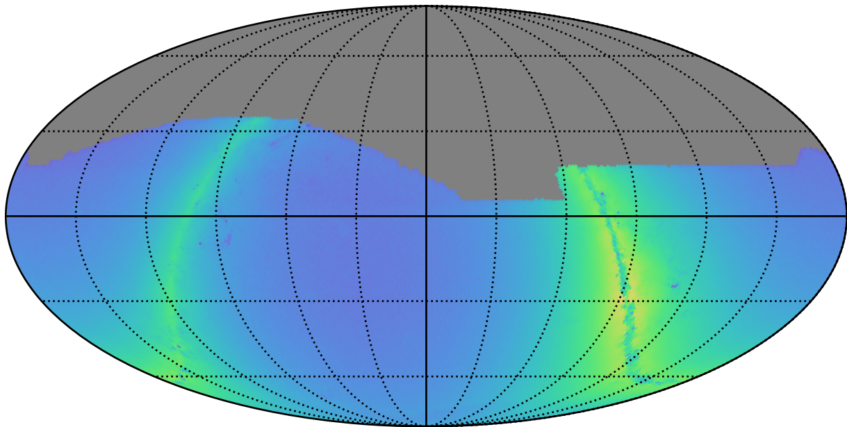
no_magell_roll_v3.4_10yrs r: Nstars_no_crowding
