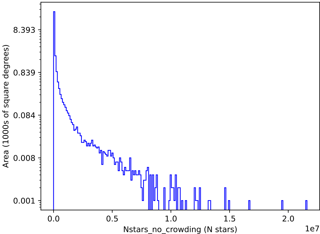
no_magell_roll_v3.4_10yrs r: Nstars_no_crowding
