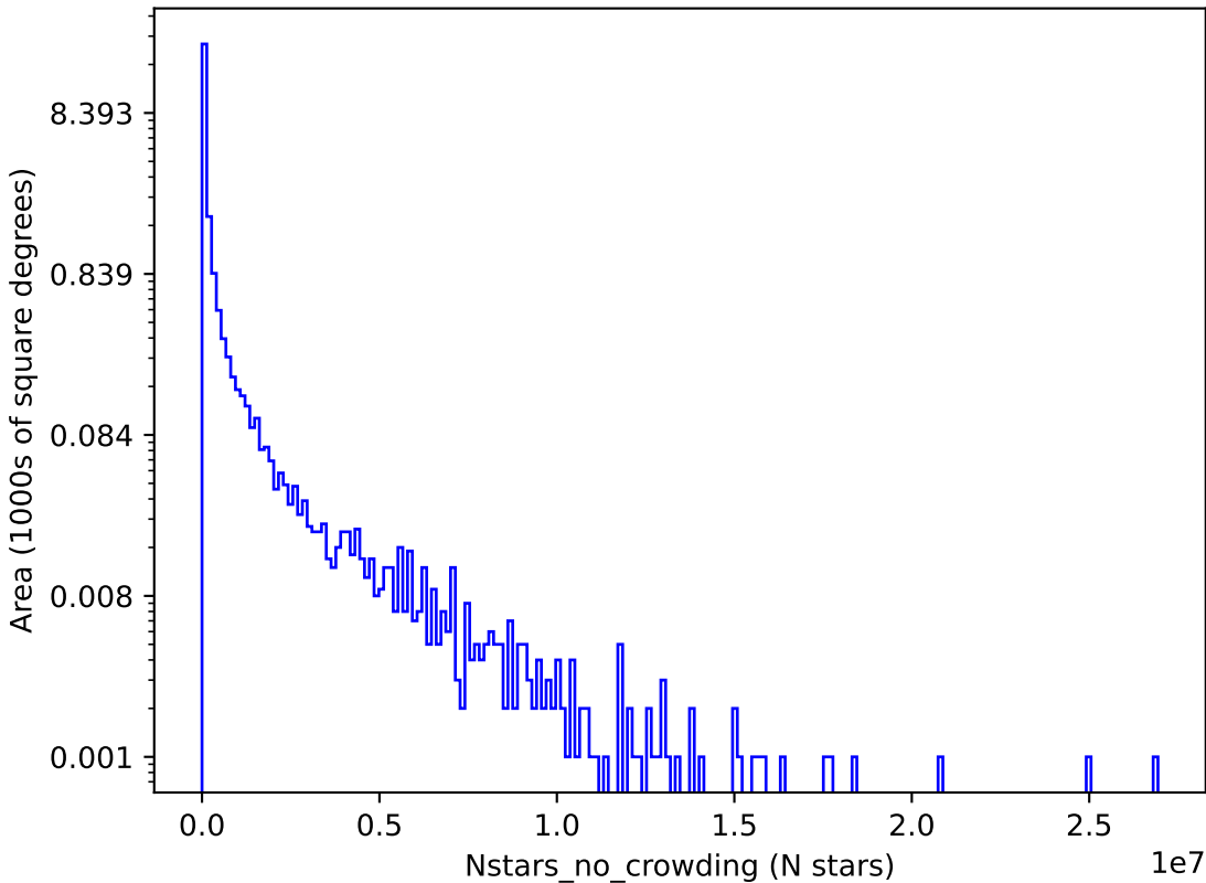
no_magell_roll_v3.4_10yrs i: Nstars_no_crowding
