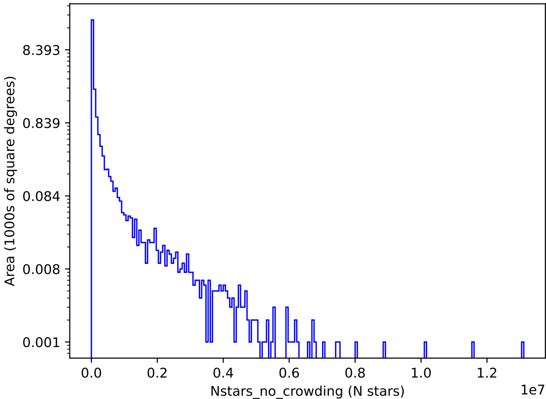
no_magell_roll_v3.4_10yrs g: Nstars_no_crowding
